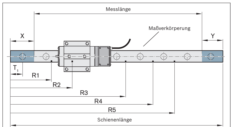
R1 ... R5 Positionen der Referenzmarken
